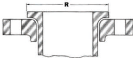
Lap-Joint
